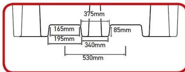
BB1DB - Passage de fourche
